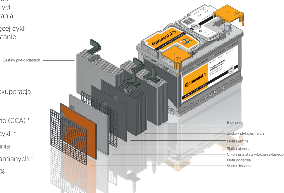
Technologia AGM: konstrukcja akumulatora
